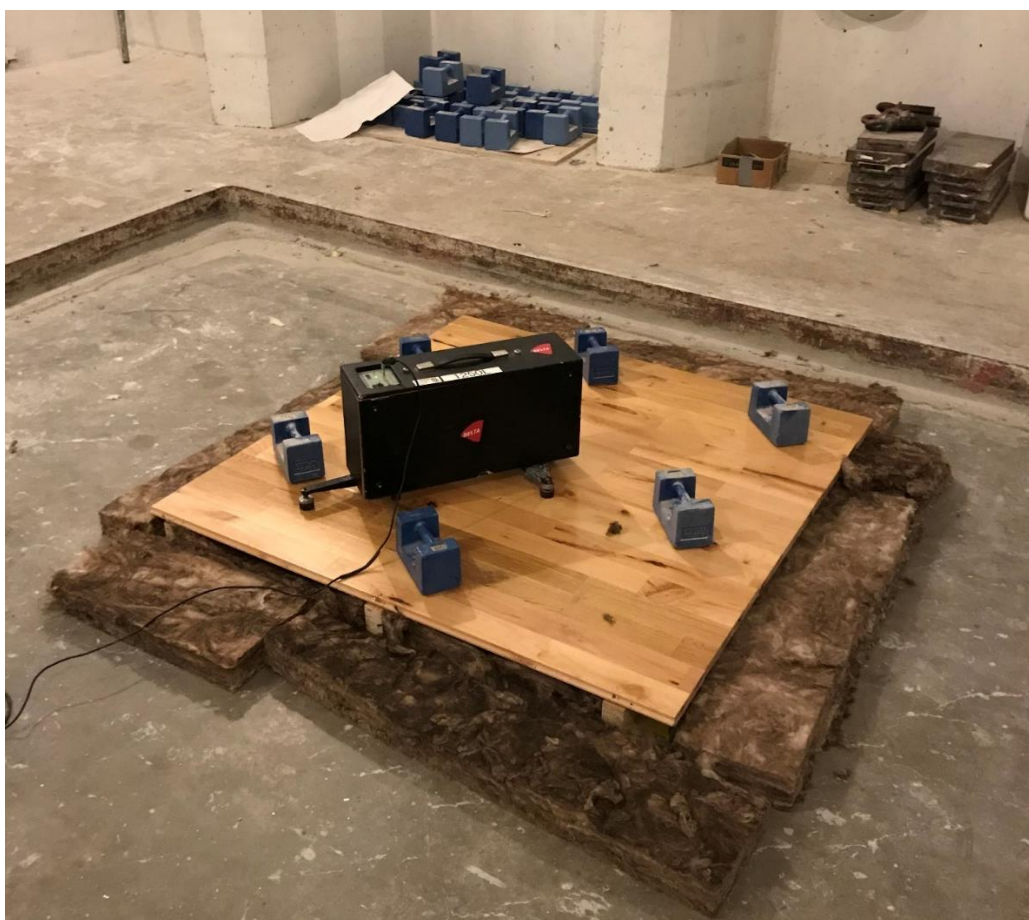
Figur 2 Foto af måleopsætningen.
